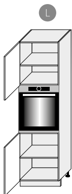
D14/RU/2D 600/2070/565
